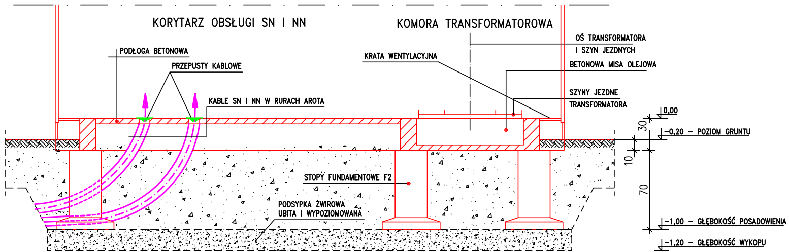
RYСУNEK PRZEDSTAWIA PRZEKRÓJ PIONOWY PRZEZ STACJĘ I POSADOWIENIE NA STOPACH BETONOWYCH TYPU F2
